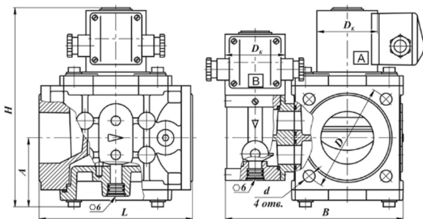
Габаритные и присоединительные размеры клапанов трехпозиционных фланцевых DN 40, 50, с двумя регуляторами расхода (давление до 0,1 МПа и 0,3 МПа)
