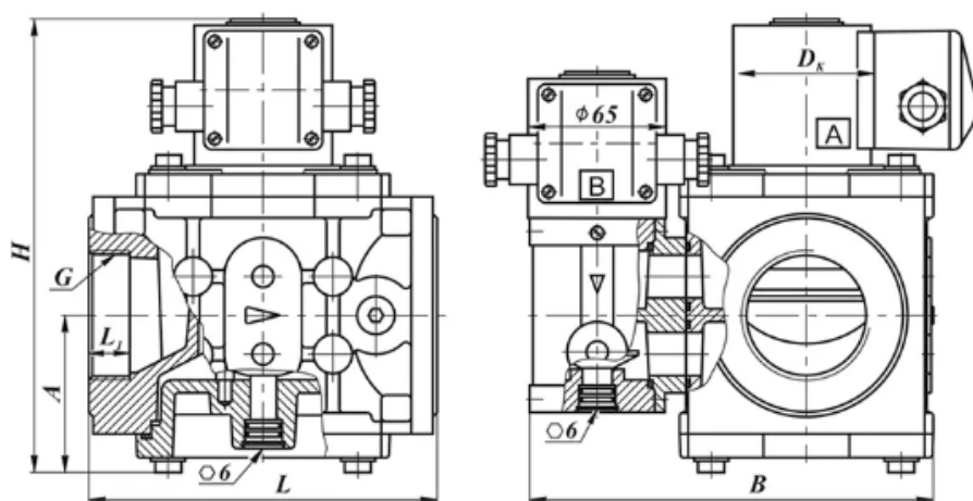
Габаритные и присоединительные размеры клапанов трехпозиционных муфтовых DN 40, 50, с двумя регуляторами расхода (давление до 0,1 МПа и 0,3 МПа)
